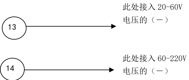
联锁控制，采用外部供电
